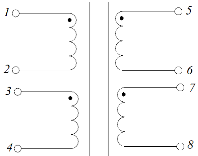
Электрическая схема
