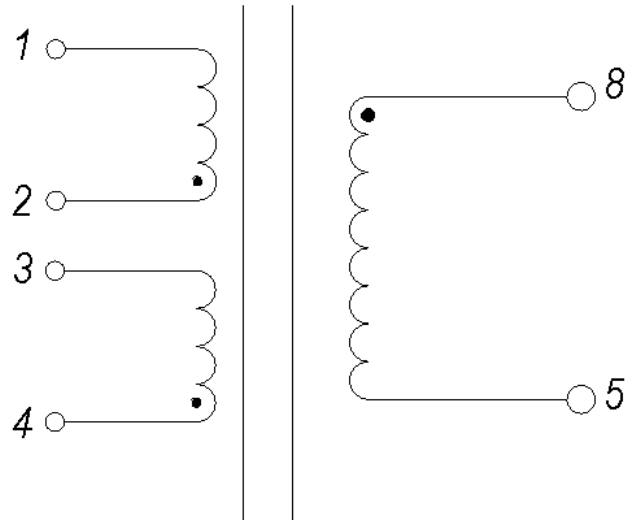
Электрическая схема
