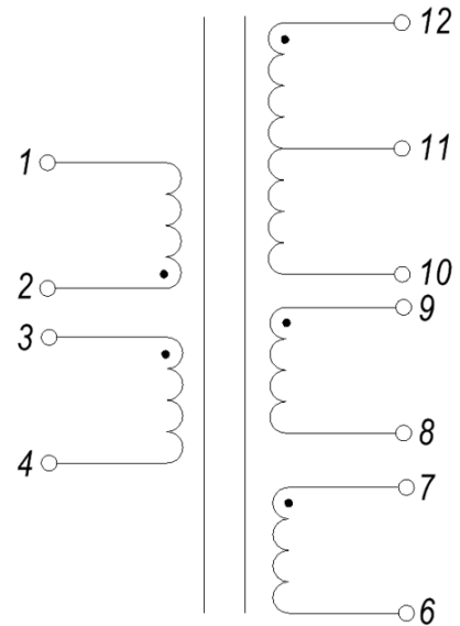
Электрическая схема
