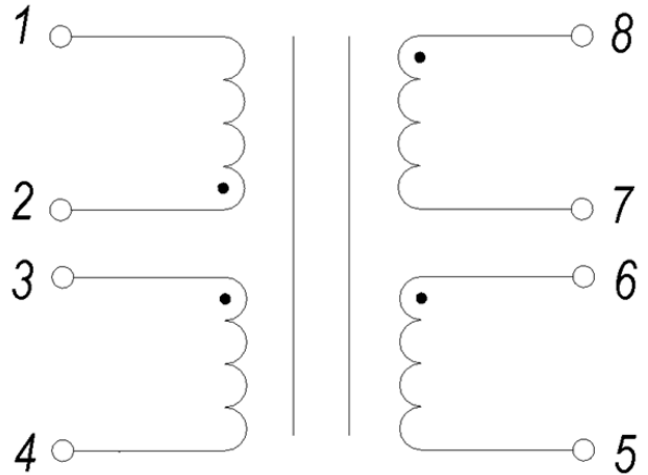
Электрическая схема
