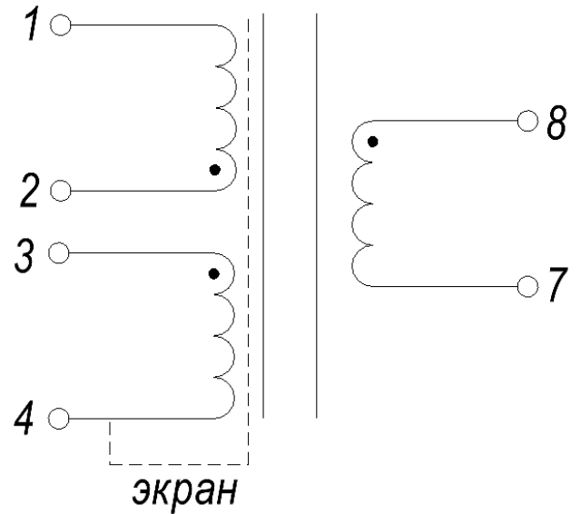
Электрическая схема
