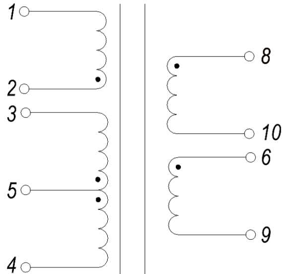
Электрическая схема
