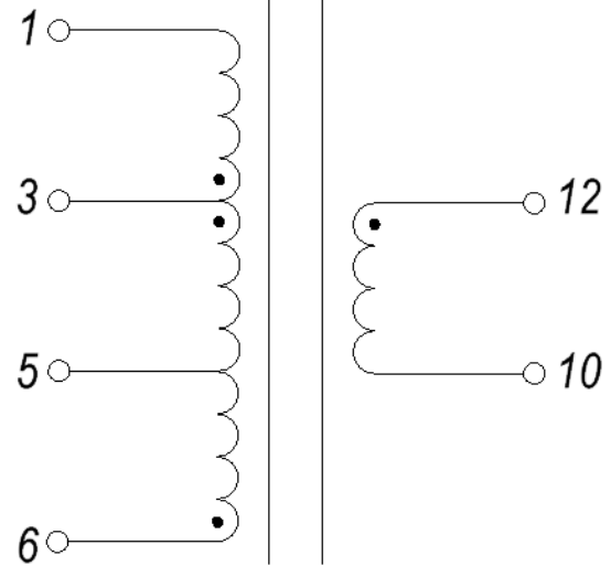
Электрическая схема
