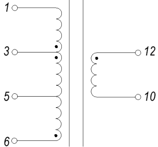
Электрическая схема
