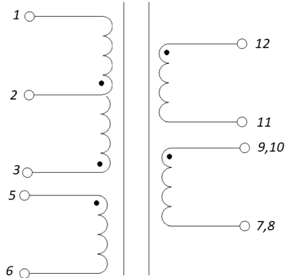
Электрическая схема
