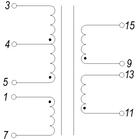
Электрическая схема
