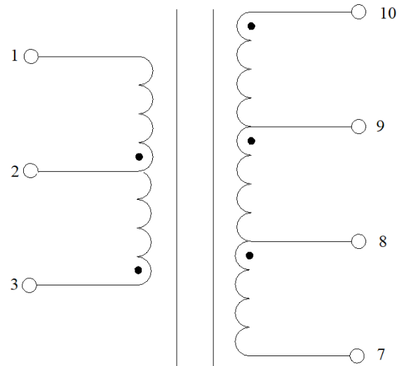
Электрическая схема
