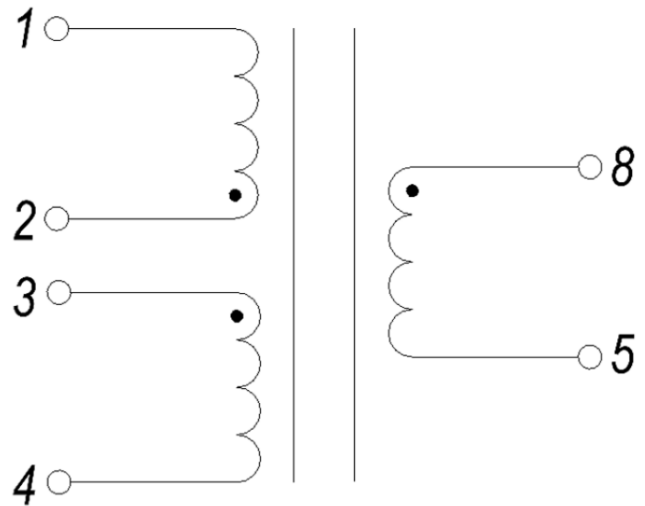
Электрическая схема
