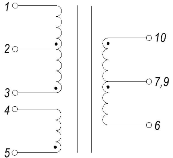
Электрическая схема
