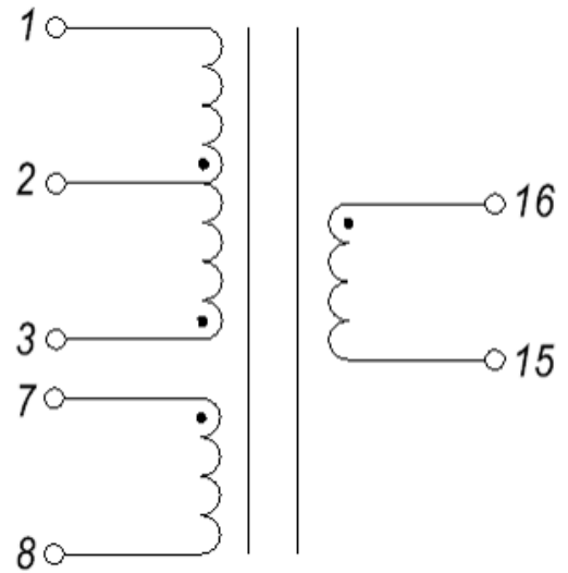
Электрическая схема
