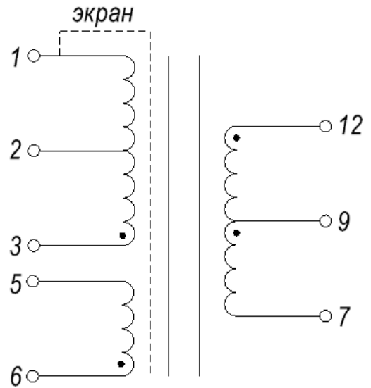
Электрическая схема
