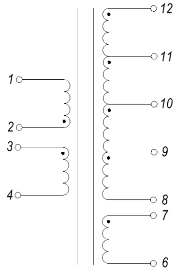
Электрическая схема
