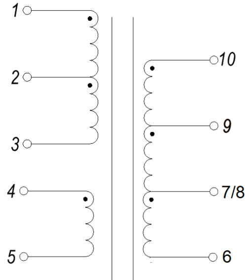
Электрическая схема
