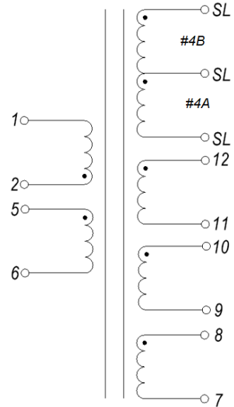
Электрическая схема
