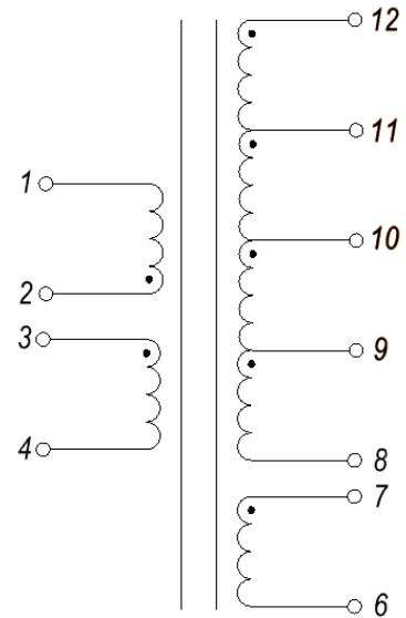
Электрическая схема
