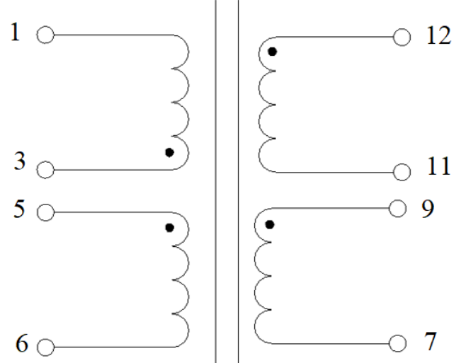
Электрическая схема
