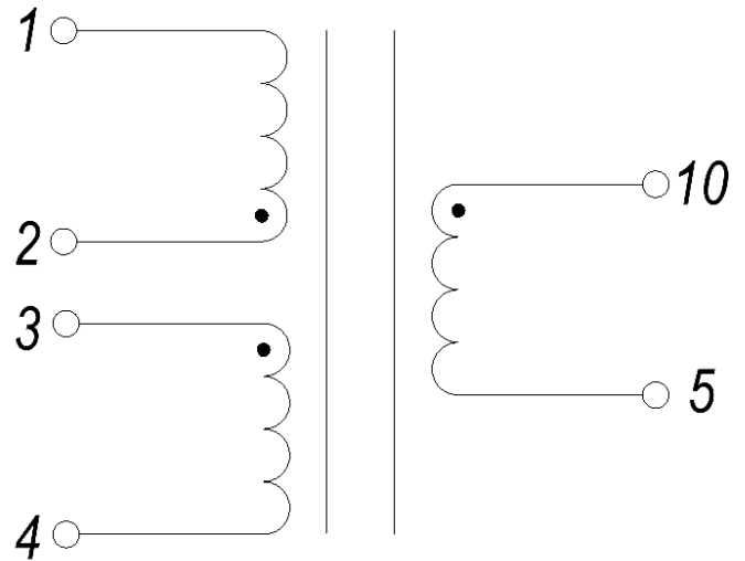
Электрическая схема
