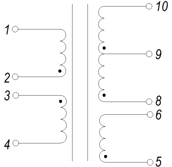
Электрическая схема
