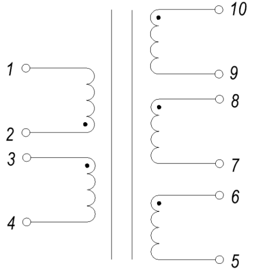
Электрическая схема
