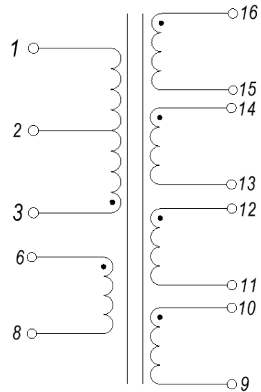
Электрическая схема
