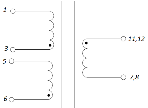
Электрическая схема
