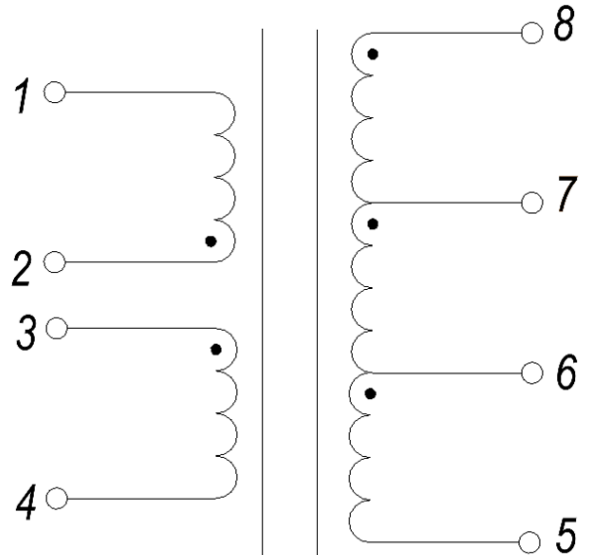
Электрическая схема
