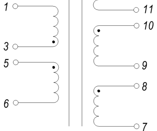
Электрическая схема
