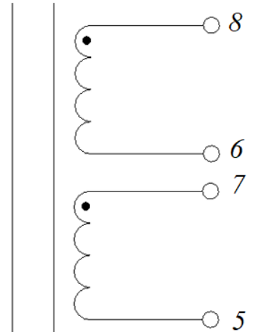
Электрическая схема
