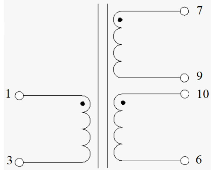
Электрическая схема
