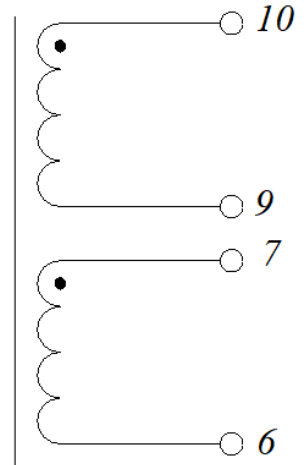
Электрическая схема
