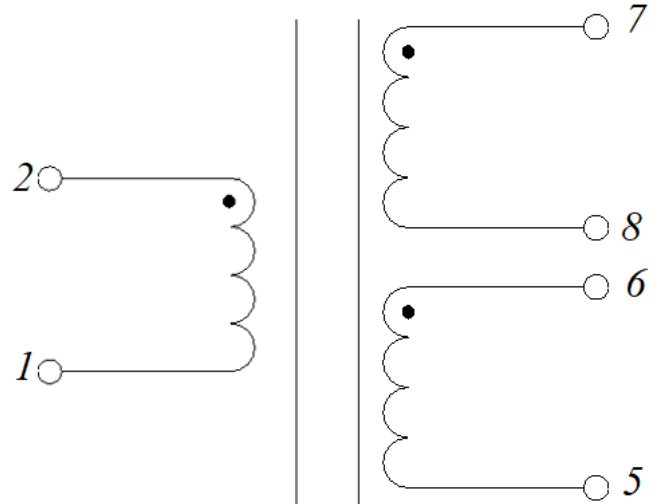
Электрическая схема
