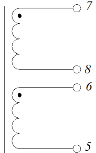
Электрическая схема
