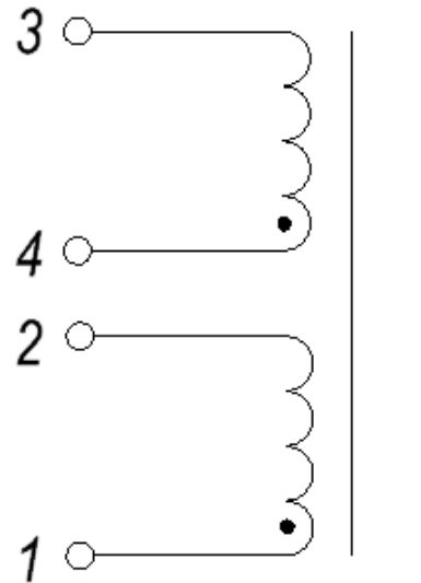
Электрическая схема
