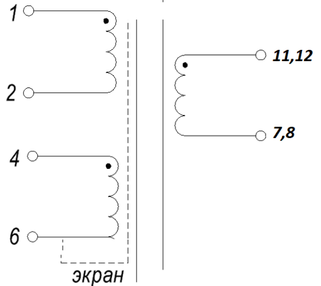
Электрическая схема
