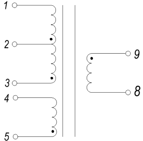
Электрическая схема
