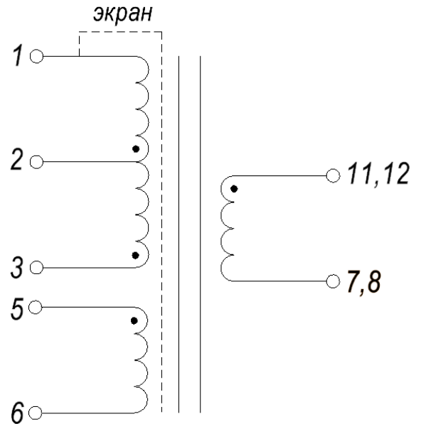
Электрическая схема
