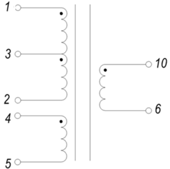
Электрическая схема
