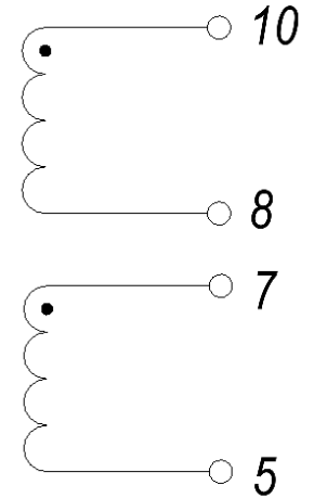
Электрическая схема
