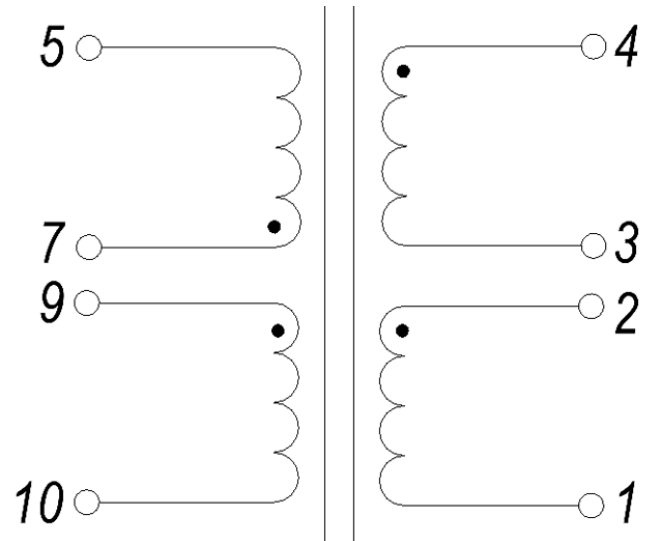
Электрическая схема
