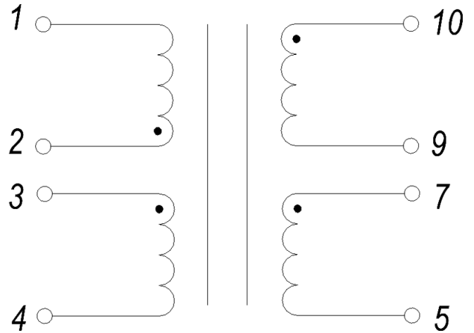
Электрическая схема
