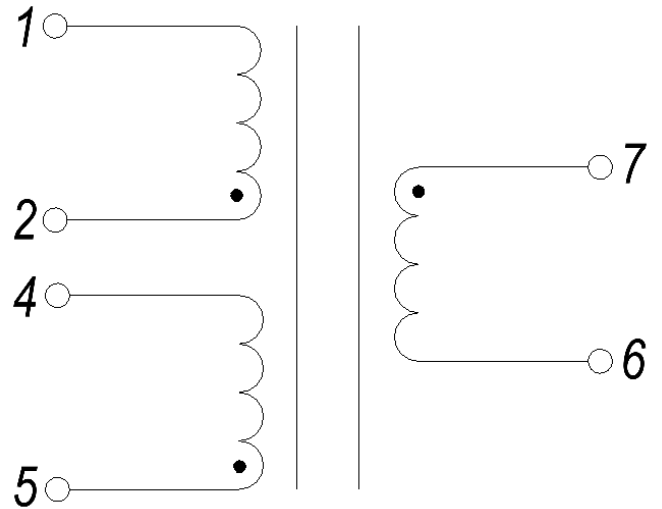
Электрическая схема
