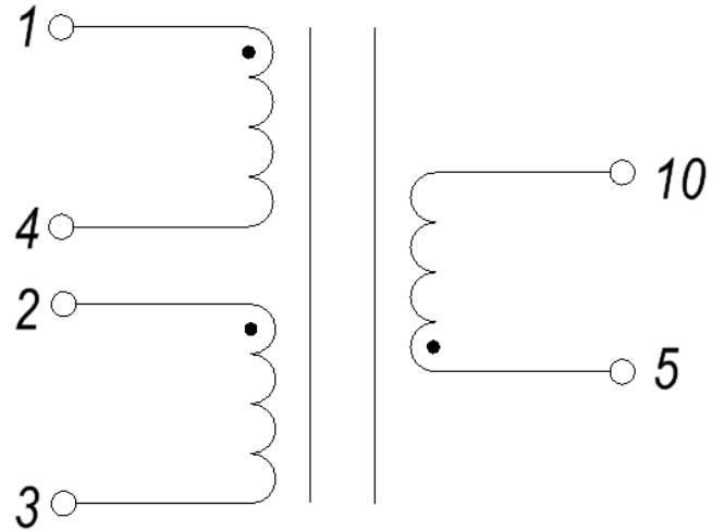
Электрическая схема
