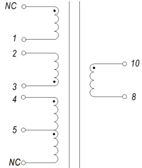
Электрическая схема
