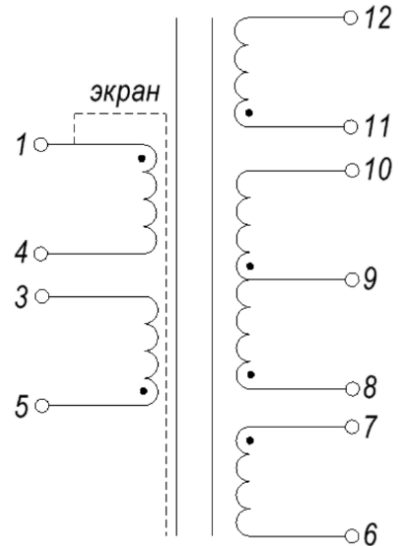
Электрическая схема
