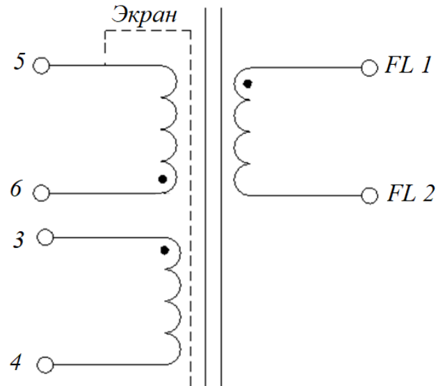
Электрическая схема
