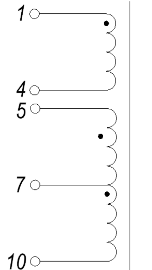
Электрическая схема
