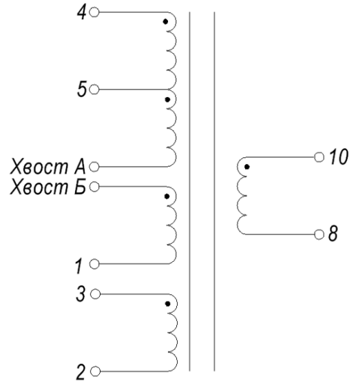
Электрическая схема
