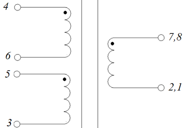
Электрическая схема
