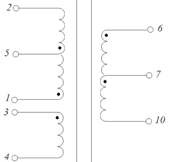
Электрическая схема
