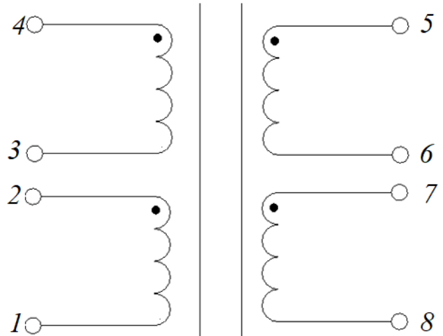
Электрическая схема
